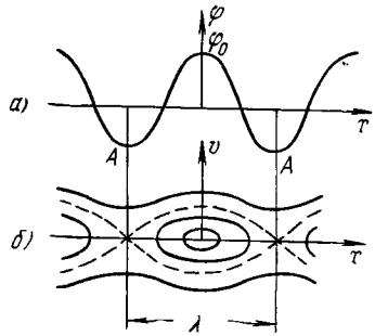
Рис. 41. Фазовые траектории электронов в волне.
