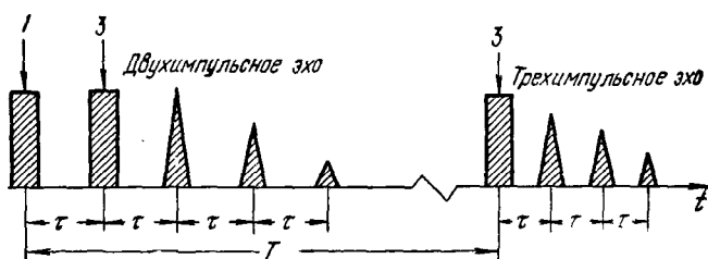
Рис. 51. Циклотронное эхо.
