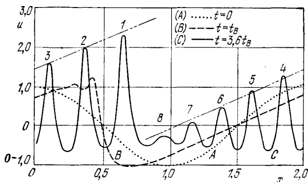
Рис. 27. Эволюция периодического возмущения в слабодиспергирующей среде [78]; t = t_B — начало опрокидывания волны.
