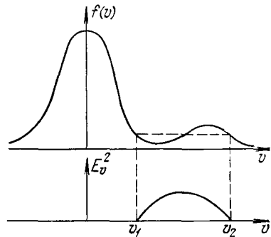
Рис. 67. Квазилинейная релаксация пучка в плазме и образование плато на функции распределения. Сплошная линия соответствует начальной, а пунктирная — конечной функции распределения. Ниже функции распределения изображено распределение энергии колебаний по фазовым скоростям после установления плато.
