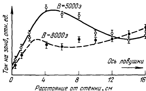
Рис. 73. Радиальное распределение плотности плазмы в ловушке.
