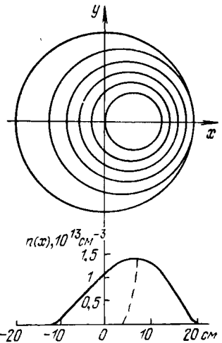
Рис. 7. Распределение плотности плазмы в установке «токамак» по сечению камеры [23].
