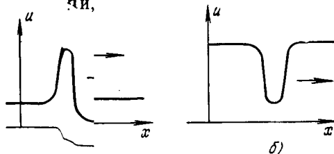
Рис. 25. Солитоны в средах с отрицательной (а) и положительной (б) дисперсией.
