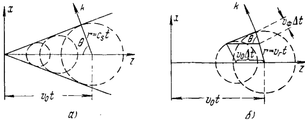
Рис. 20. Сложение волн от движущегося источника в среде без дисперсии (а) и с дисперсией (б).
