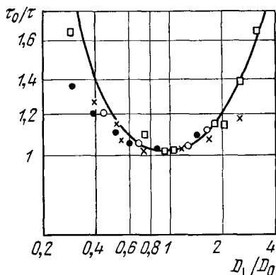
Рис. 10. Время жизни распадающейся плазмы в тороидальной трубке (газ — гелий, R = 28 см, a = 0,3 см) при давлениях: 0,025 ( \bullet ), 0,04 ( \circ ), 0,055 ( \times ), 0,12 ( \square ) мм рт. ст.
